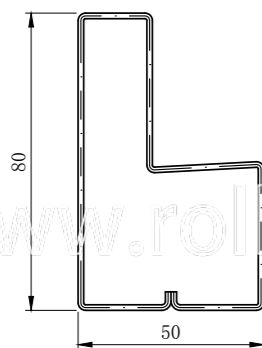
辊压厚度: 1.5-2.0mm Rolling thickness: 1.5-2.0mm 辊压材料: G340-G550镀锌板、冷轧板 Rolling material: G340-G550 galvanized sheet, cold rolled sheet
