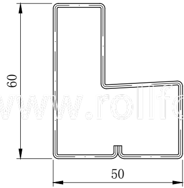
辊压厚度: 1.5-2.0mm Rolling thickness: 1.5-2.0mm 辊压材料: G340-G550镀锌板、冷轧板 Rolling material: G340-G550 galvanized sheet, cold rolled sheet
