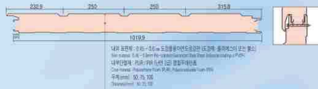
볼트레스 500골 Boltless 500 corrugations panel
